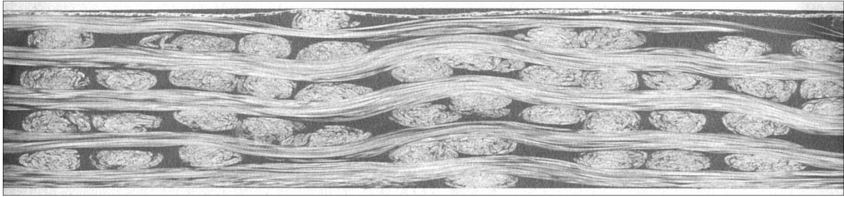
Fig. 1: Tissage interlock 3D non-injecté et non-compacté
